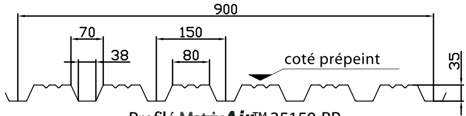
Profilé MatrixAir™ 35150-BR
